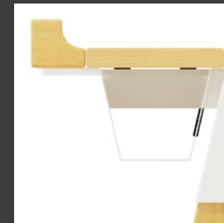
Abschlussleiste und Unterbau End profile and substructure
