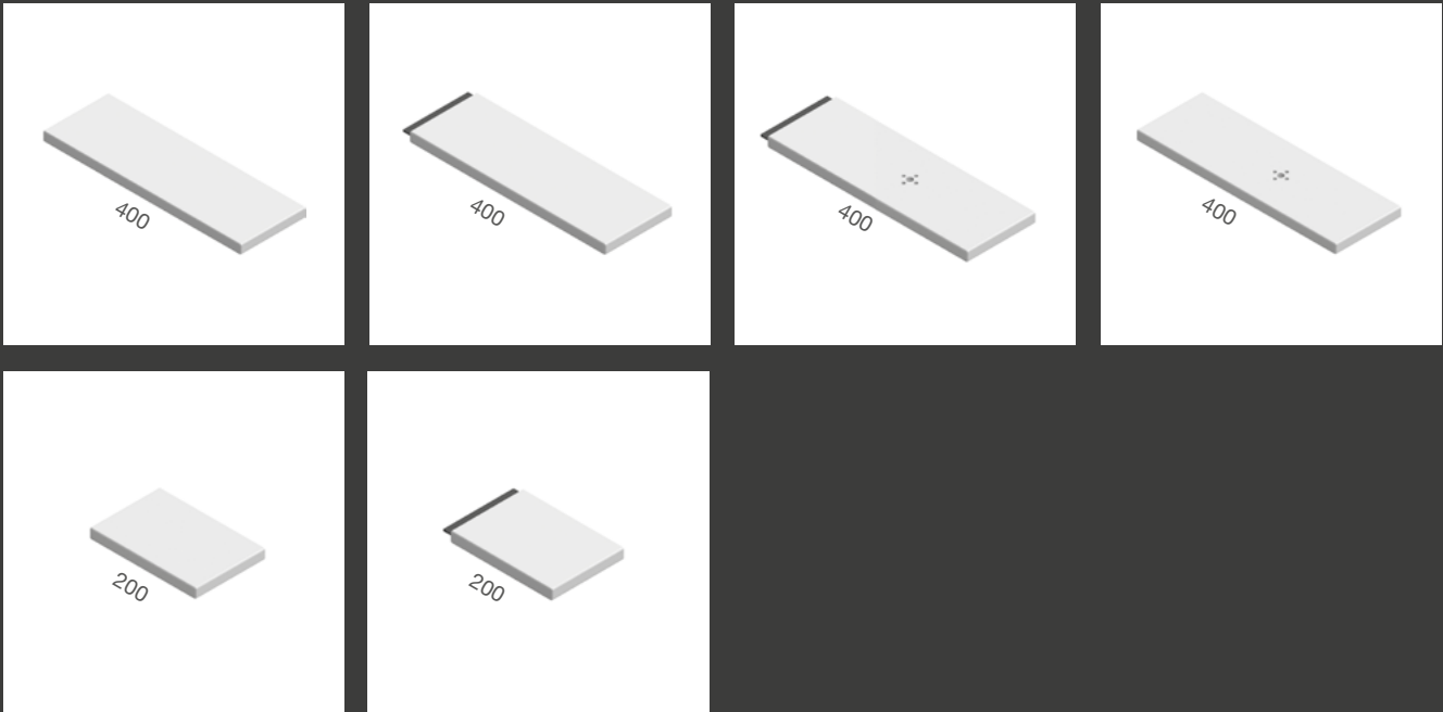
Einsätze Dekorplatte / mit Bürste als Kabeldurchlass / mit Bürste und Bohrung für Monitorhalter / mit Bohrung für Monitorhalter Inserts decor panel / with brush as cable aperture / with brush and hole for monitor holder / with hole for monitor holder
