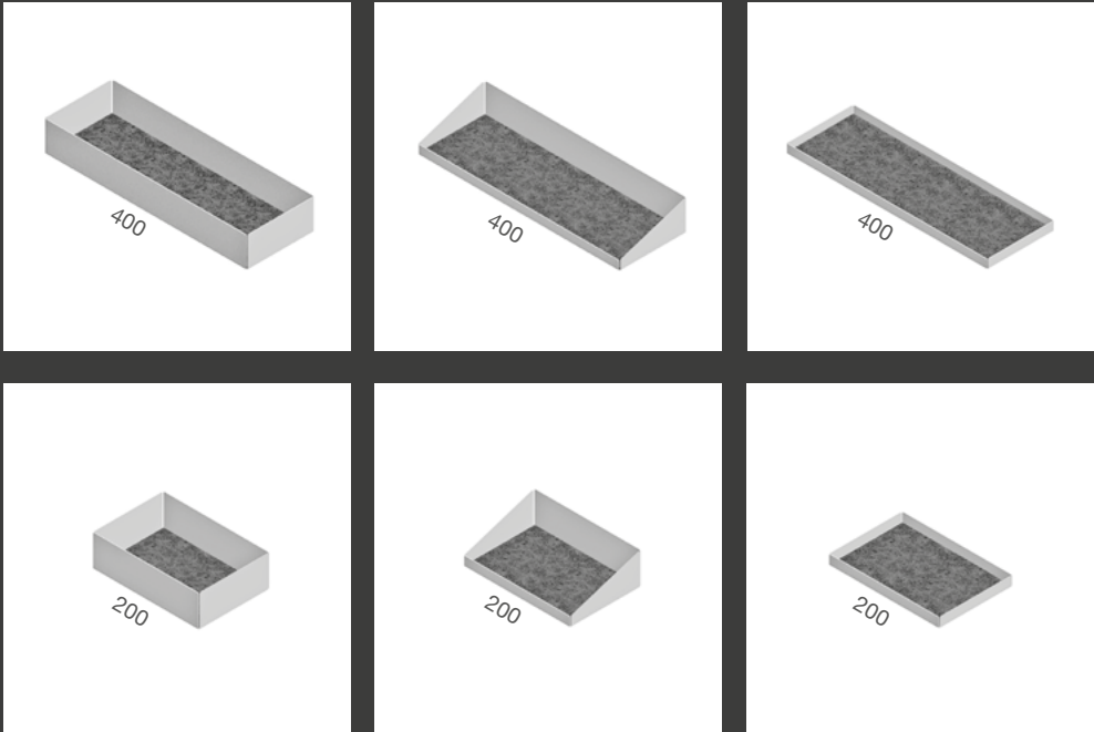
Einsätze aus Blech mit Filzeinlage hoch / ansteigend / flach Sheet metal inserts with felt insert high / rising / flat
